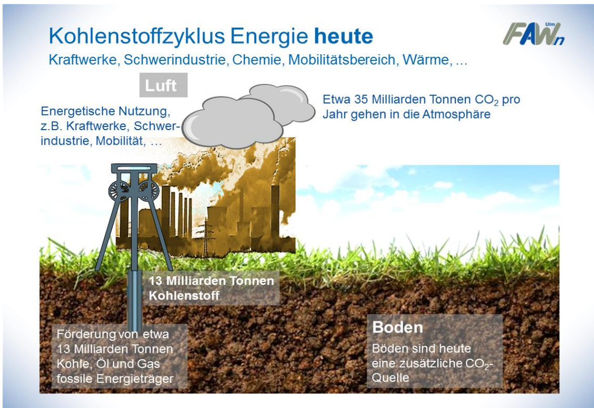
Abb. 4 Heutiger Kohlenstoffzyklus
